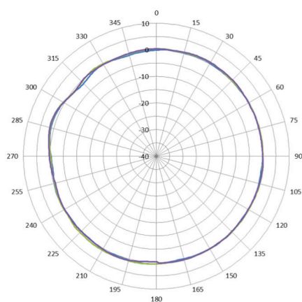
H-plane – 2.4 GHz
