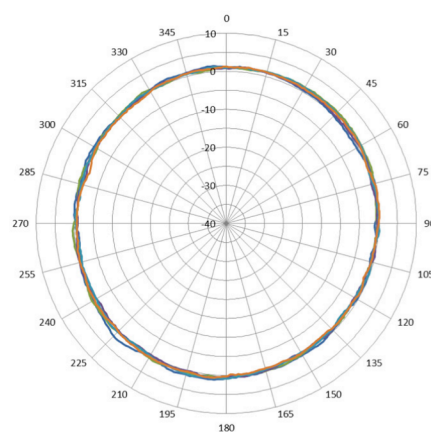
H-plane – 5 GHz
