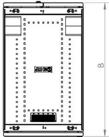
Ansicht von oben (600 mm Breite)
