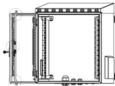
3-Punkt-Verriegelungssystem
