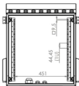
Innenansicht
