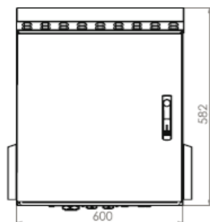
Frontansicht
