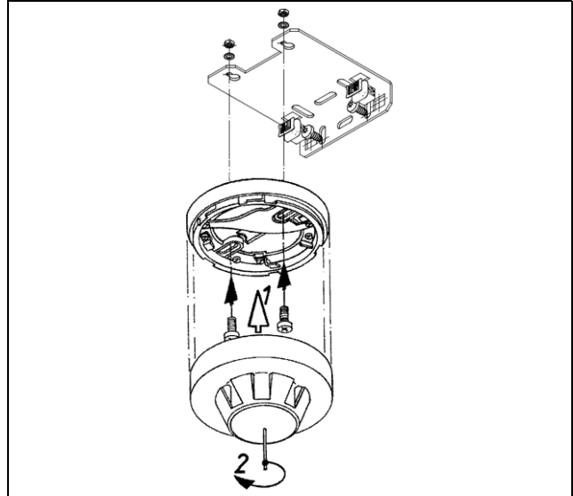
Abb. 2: Montage des Rauchmelders
